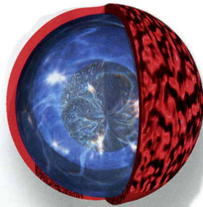
Het West-Nijlvirus
